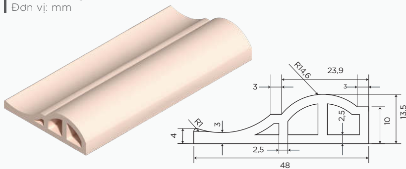
Phào chỉ rỗng Đơn vị: mm
